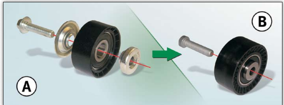
Rolka prowadząca 532 0433 10, wersja stara (A) i nowa (B)
